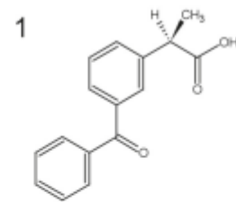
Ketoprofen (MW 254.3)
