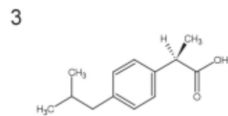
Ibuprofen (MW 206.3)
